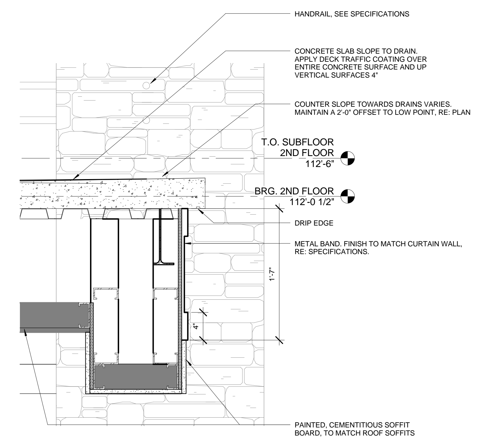
2 TERRACE EDGE AT TOWN CENTER SCALE: 1 1/2" = 1'-0"
