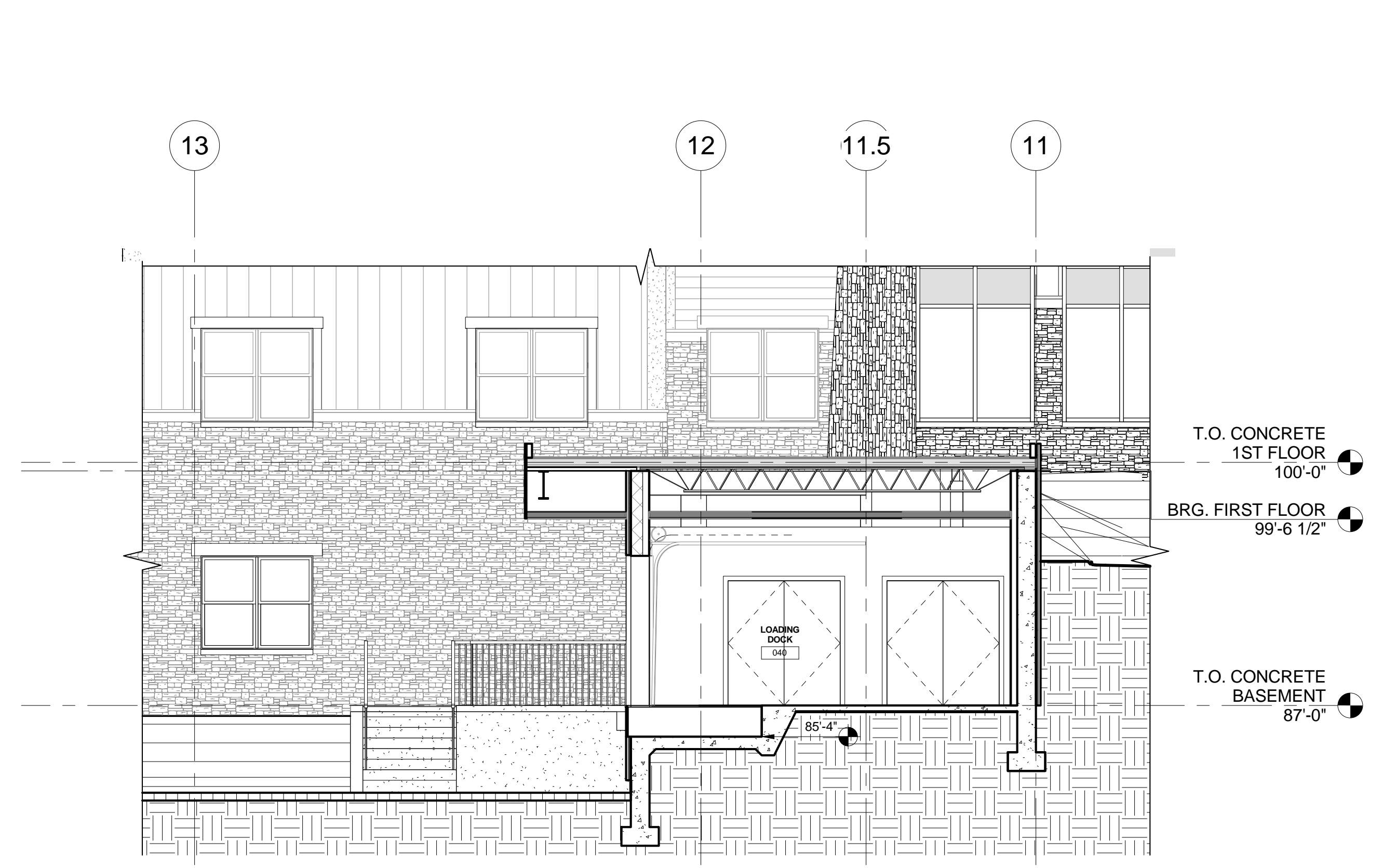
E BLDG. SECTION E SCALE: 3/16" = 1'-0"
